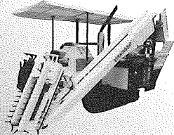
自走式 大根収穫機 HD1400 【1条幅】
